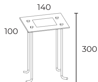
Закладная деталь H=300 мм
